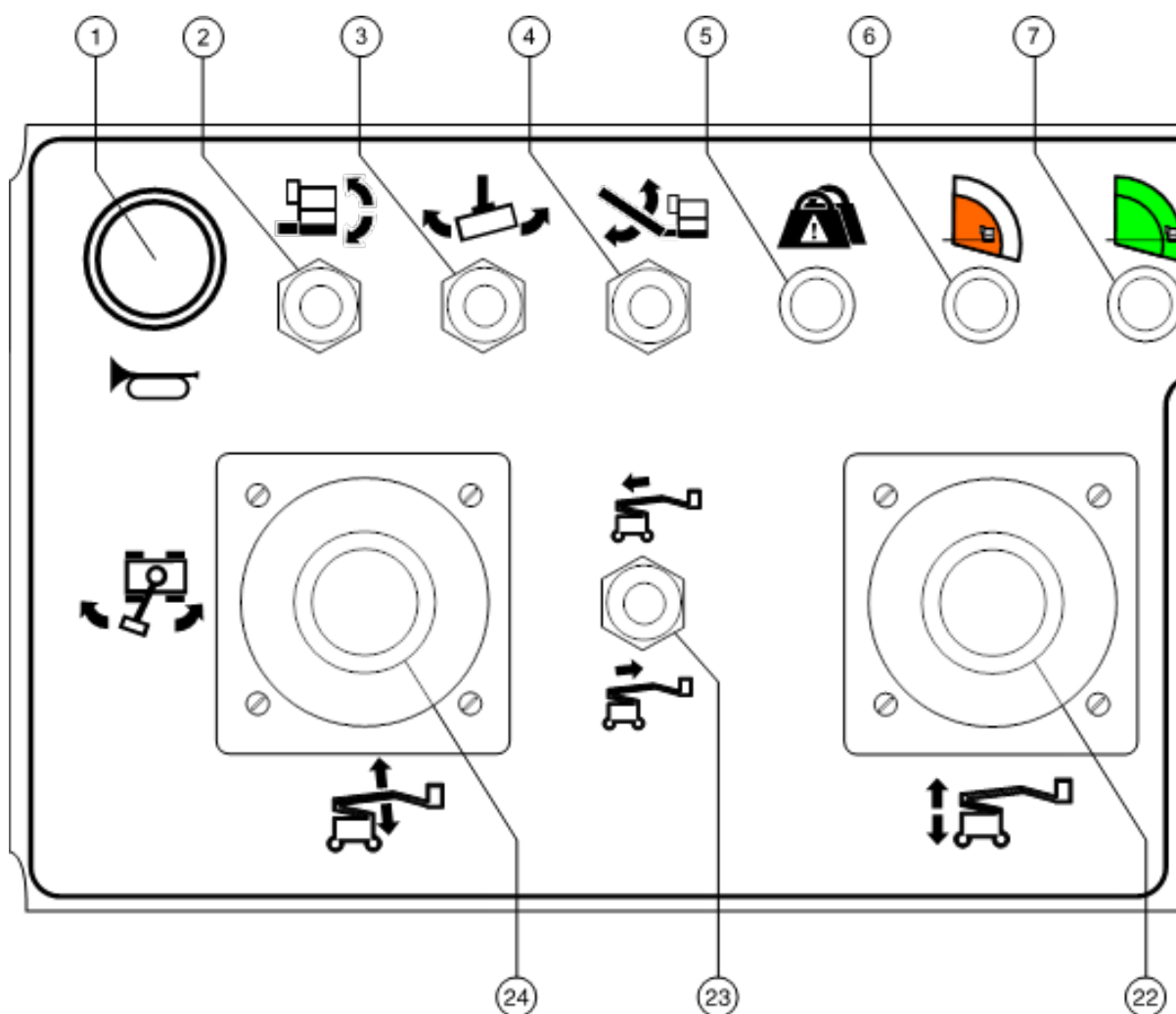
Platformsbetjeningspanel med timetæller
