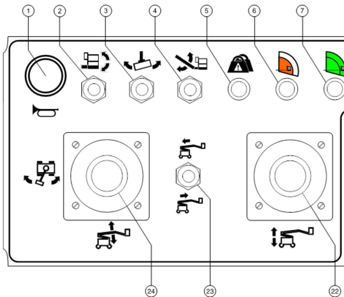
Platformsbetjeningspanel med LCD-skærm
