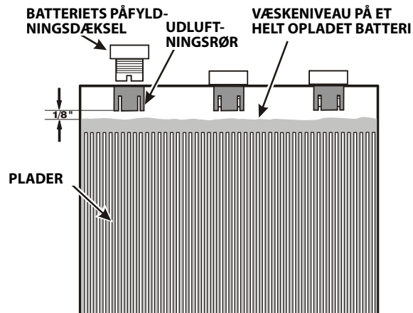
Figur 6-2. Batterivæskenniveau
