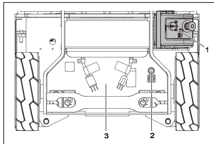
Figur 4-17. Elektrisk bremseudløsning
