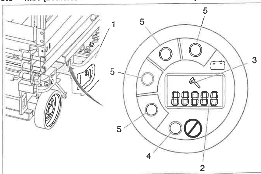
Figur 3-4. MDI (Digital multifunktionsindikator)
