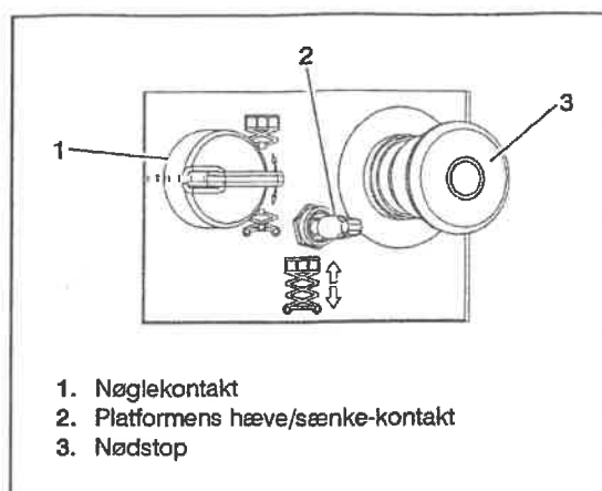
Figur 3-1. Undervognens styrepanel
