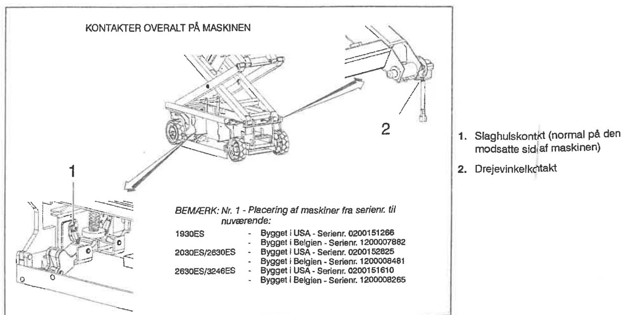
Figur 2-5. Placering af kontakter - 2 af 2
