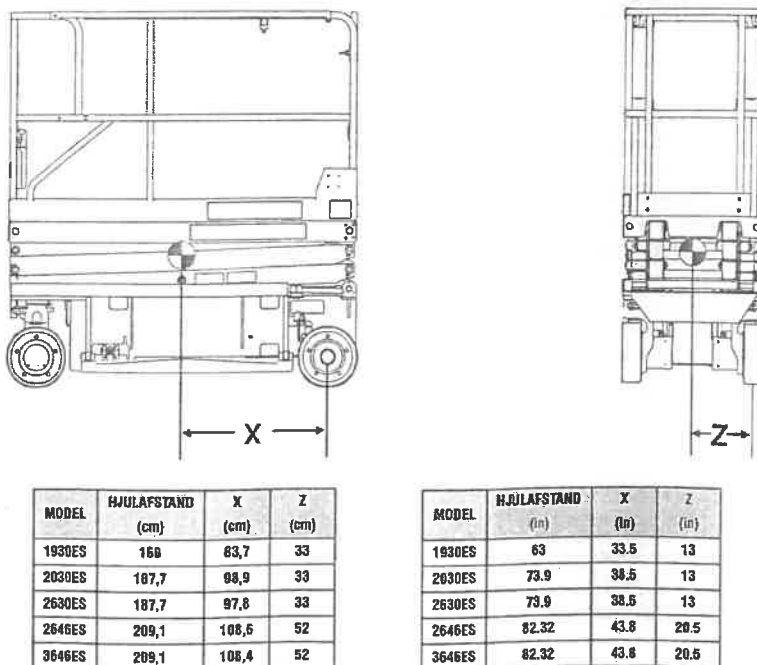
Figur 4-4. Skema over løftning og fastspænding
