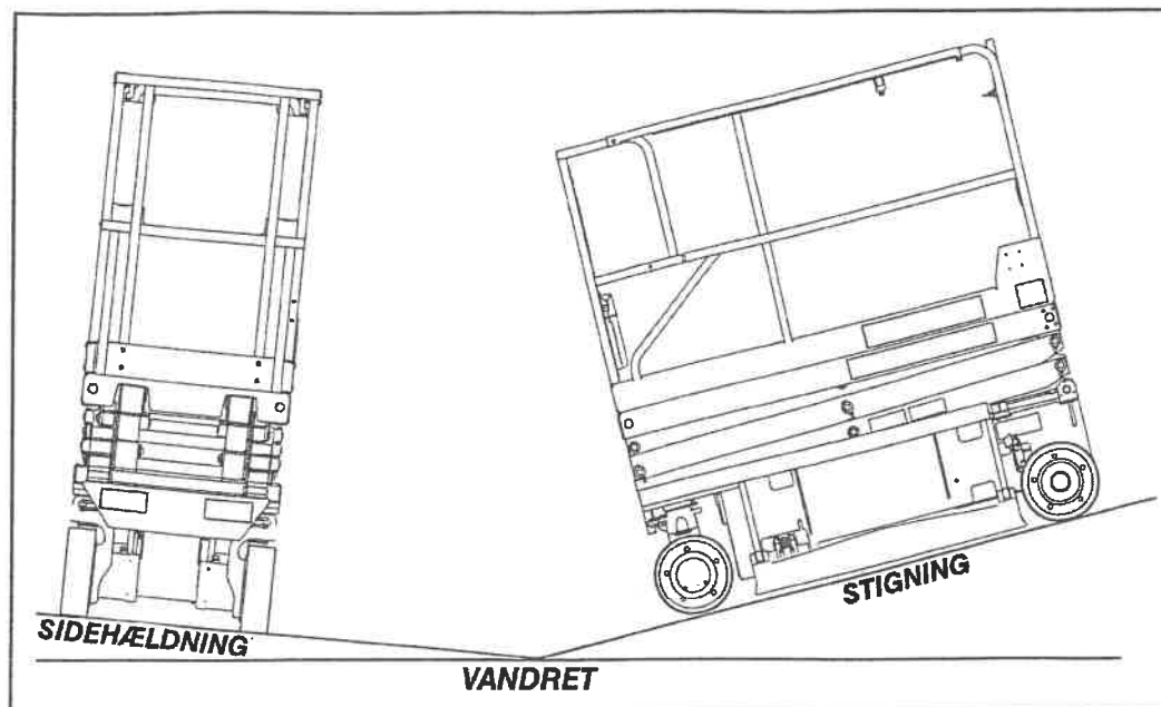
Figur 4-1. Stigning og sidehældning
