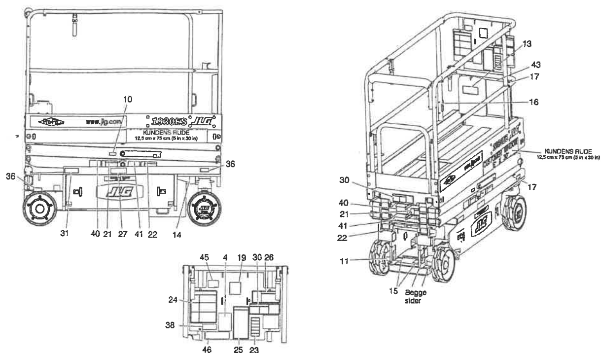
Figur 3-5. Placering af mærkater - 1930ES - Blad 2 af 2
