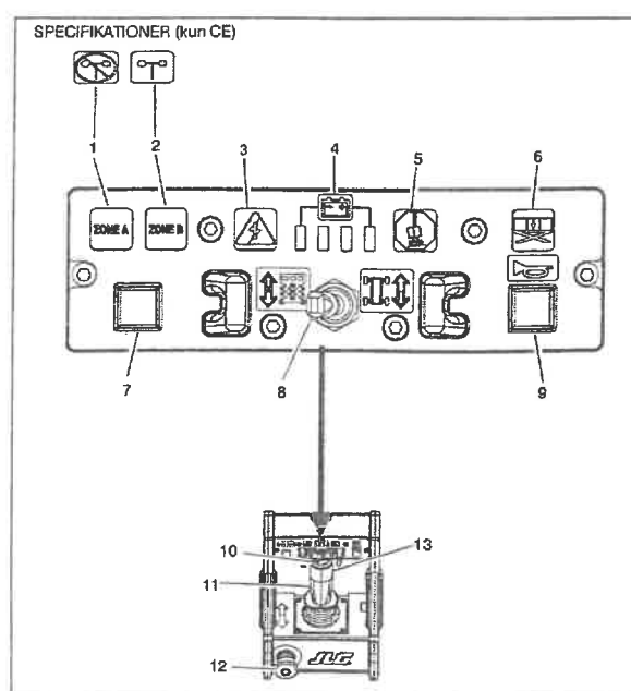
Figur 3-3. Plattformens styrepanel
