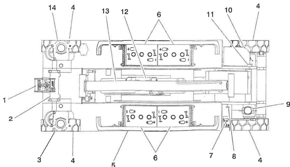
Figur 2-1. Daglig inspektion ved rundgang - Blad 1 af 3
