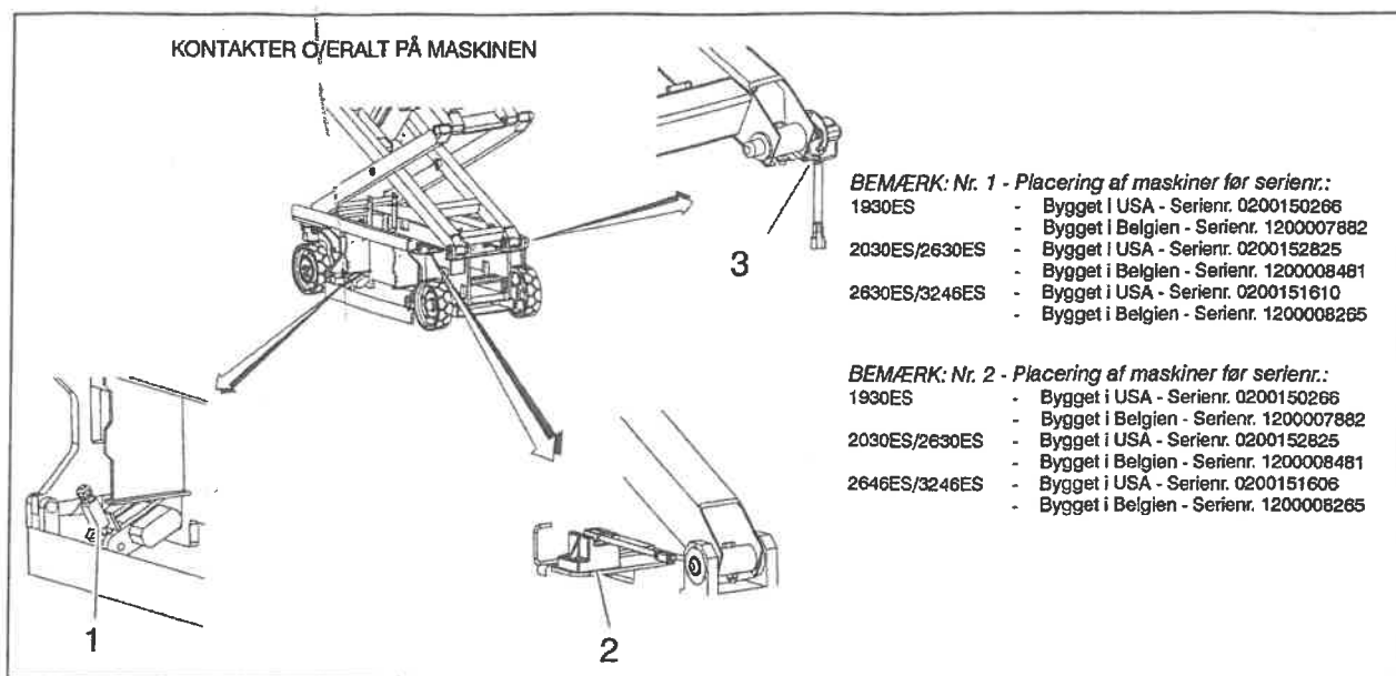
Figur 2-4. Placering af kontakter - 1 af 2
