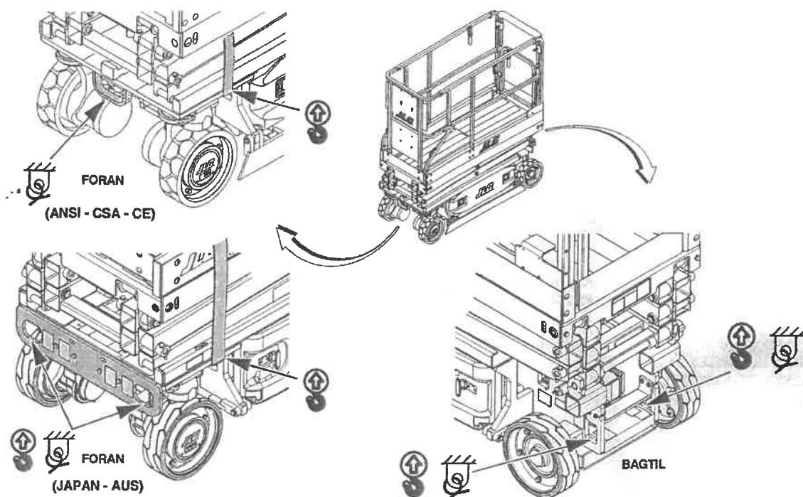
Figur 4-2. Diagram over løftning og fastspænding
