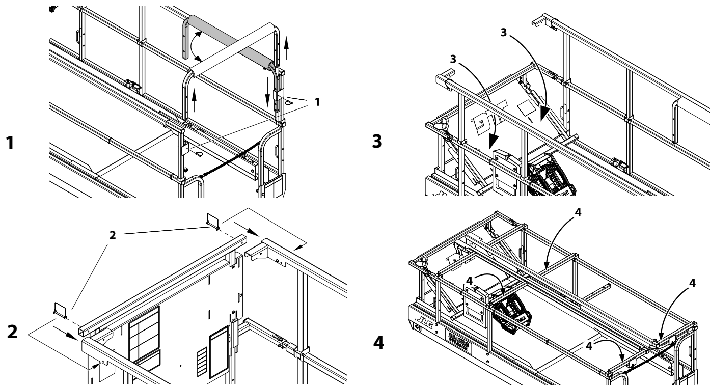
Figur 3-6. Platformens gelændere – Nedfoldningssekvens
