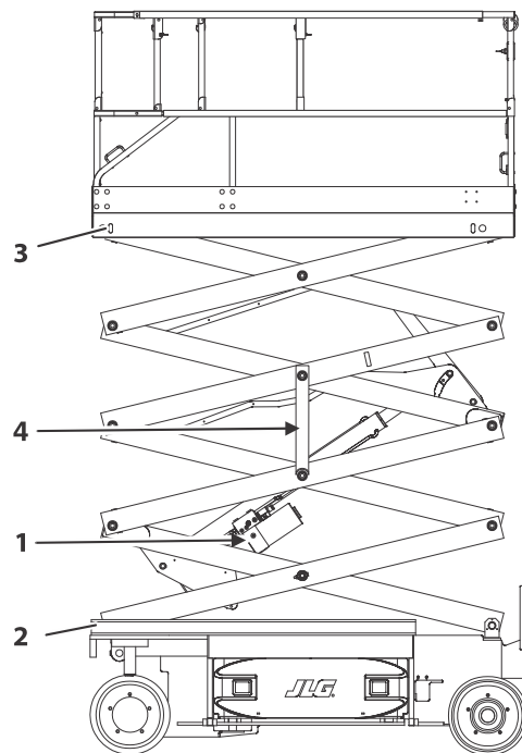
Figur 6-1. Smøreskema
