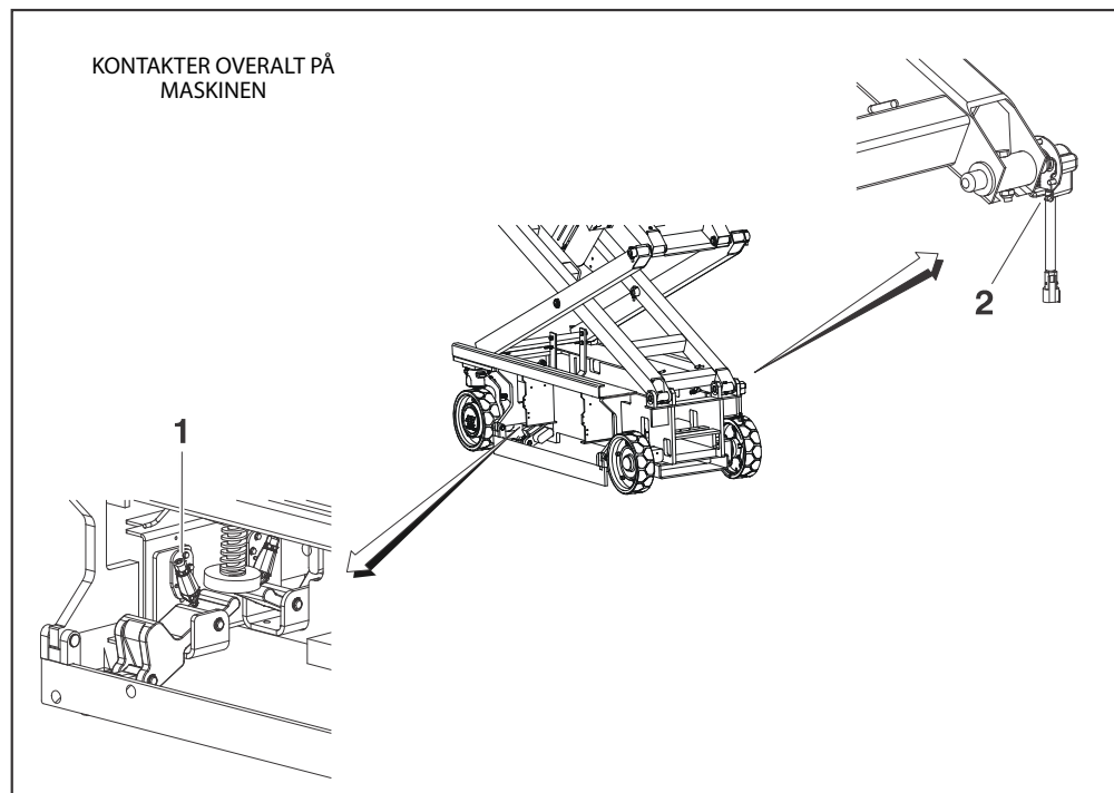
Figur 2-1. Kontaktplaceringer
