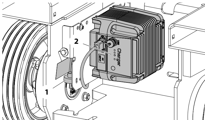
1. Kabel til vekselstrømsstik 2. Opladningsindikatorens LED'er
