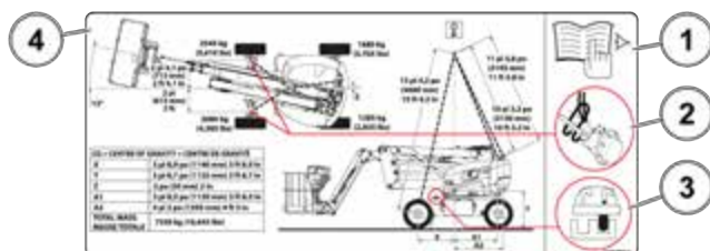
Figur 39: Mærkat - Ved løft
