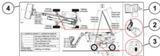
Figur 38: Mærkat - Ved løft
