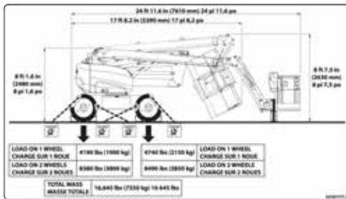
Figur 37: Mærkat - surring
