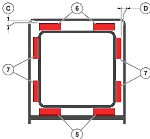
Figur 200: Kontrol af afstandsstykket på teleskoparmen 5 - 160 ATJE S1 - 160 ATJE RC S1
