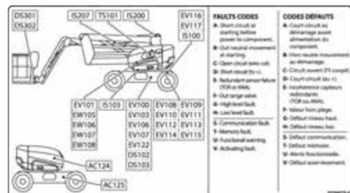
Figur 32: Mærkat - Fejlkode
