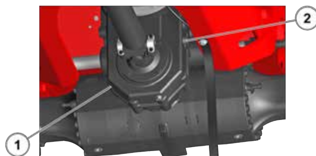
Figur 148: Kontrol af reduktionsgearet for lækager
