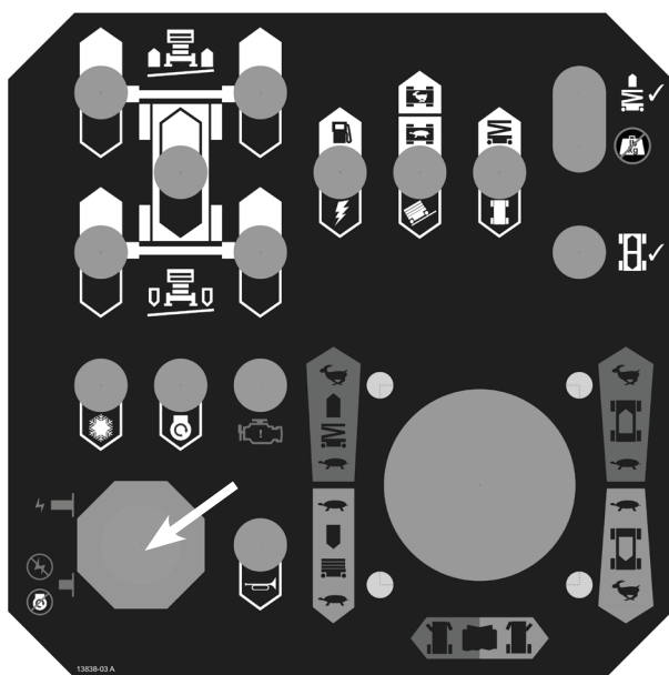
Figur 4.1 - Øvre kontroller i nødsituation Stopkontakt
