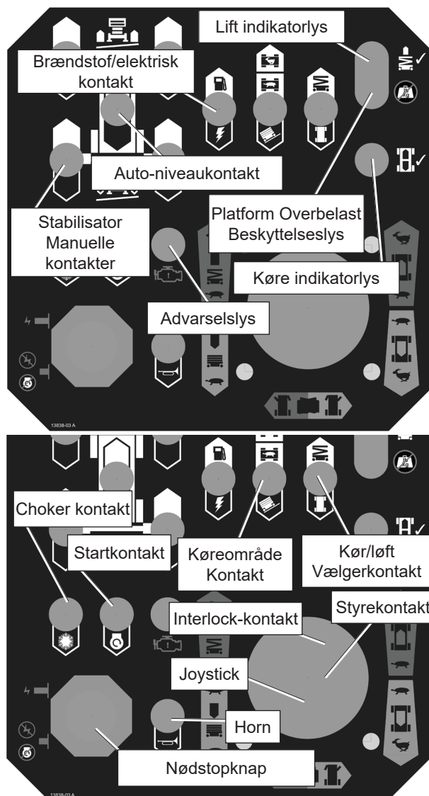
Figur 6.3 - Øvre kontroller
