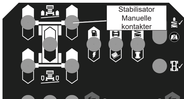
Figur 8.5 - Stabilisator manuelle kontakter:
