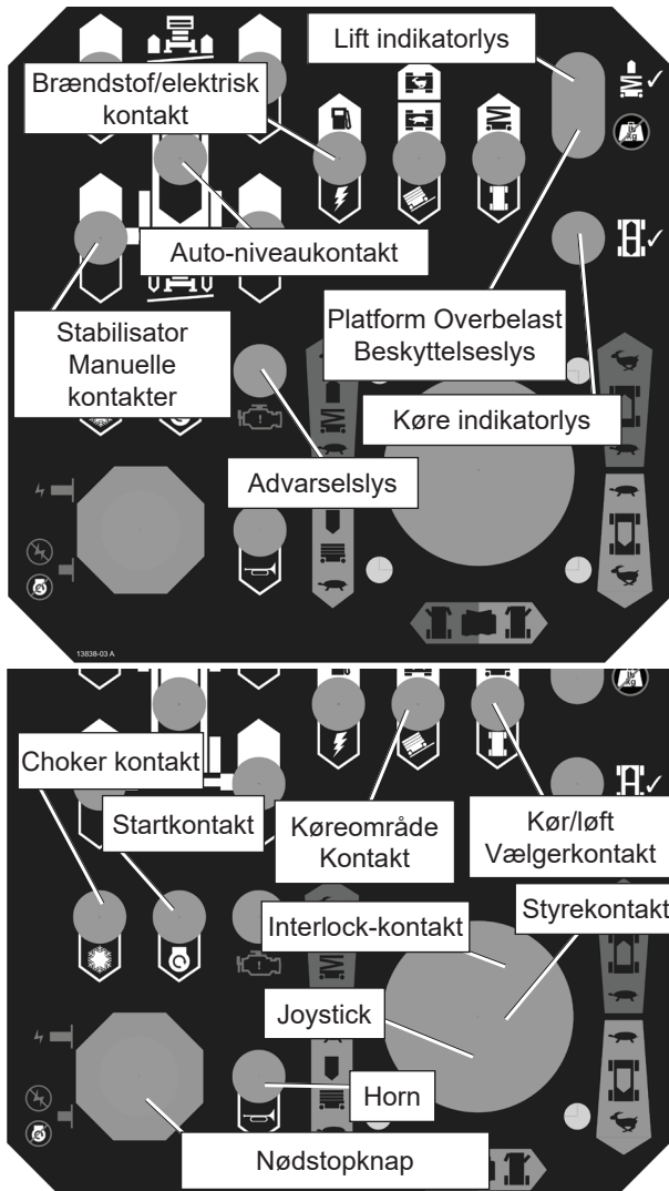
Figur 8.2 - Øvre kontroller
