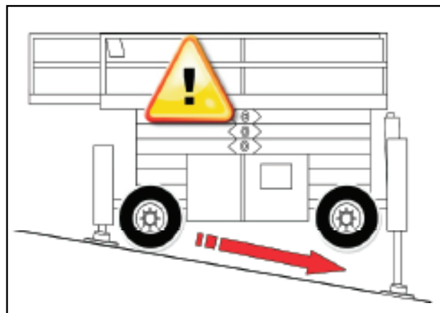
Figur 8.12 - Maskine på skråning
