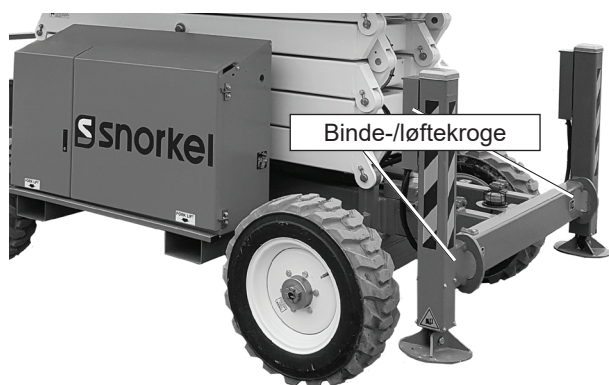
Figur 9.4 - Løfteskrogpunkter
