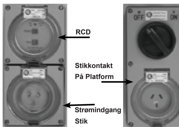
Figur 4.13 – RCD/ELCB AC Stikkontakt
