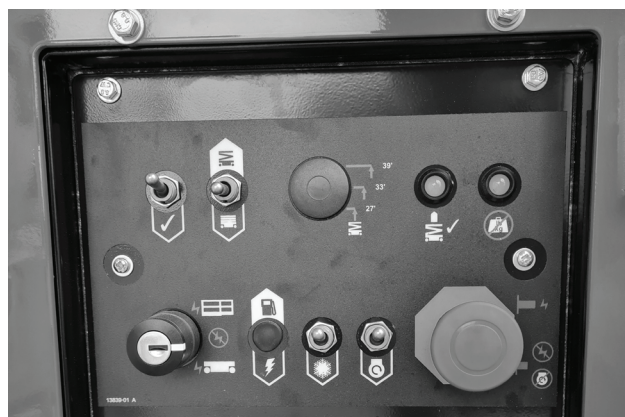
Figur 7.7 - Nedre kontroller
