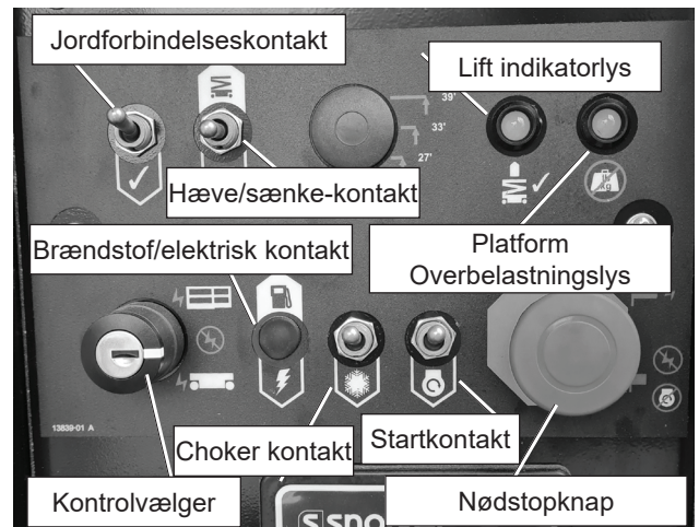
Figur 6.2 - Nedre kontroller
