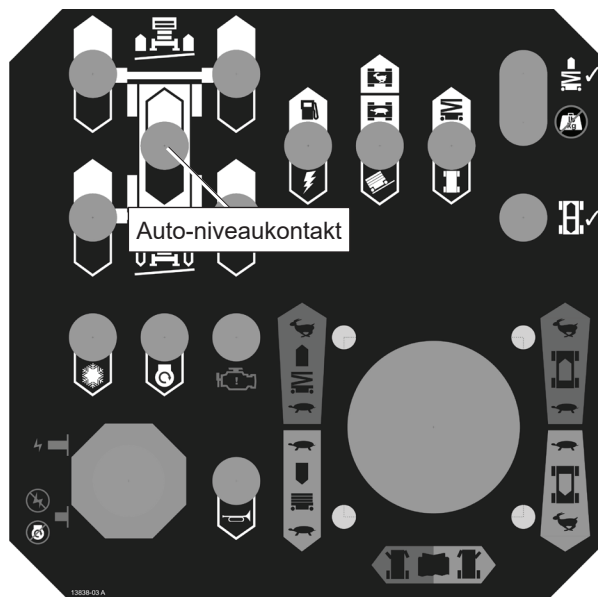
Figur 8.9 - Automatisk niveaukontakt
