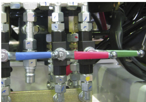
Fig. 35d Nødsænkingsventiler
