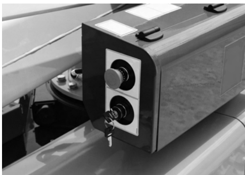
Fig. 60 Nødstopknapp på bælte
