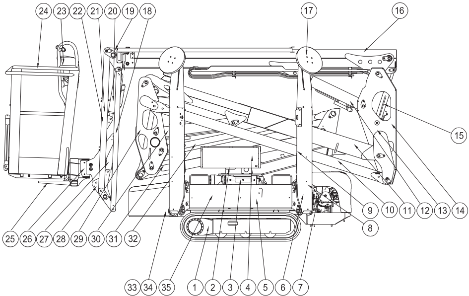
Fig. 5 Terminologi for maskinens komponenter
