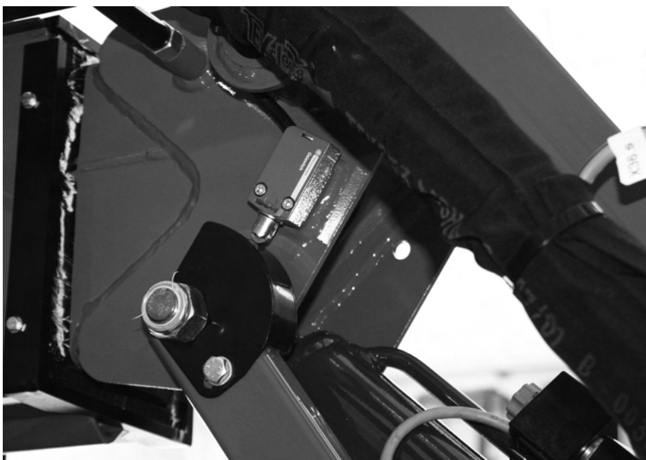
Fig. 16 Mikrokontakt til kranarm
