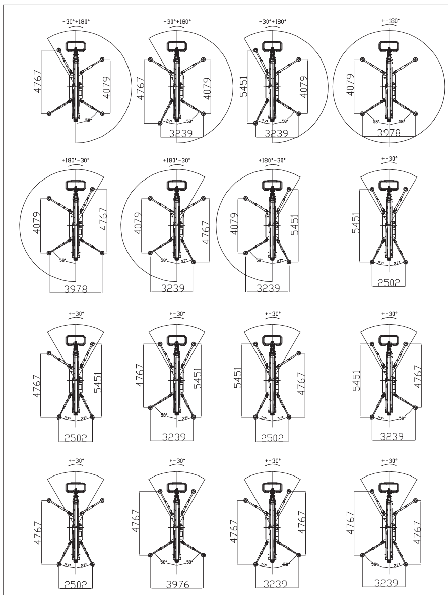
Fig. 97 Stabiliseringsområder
