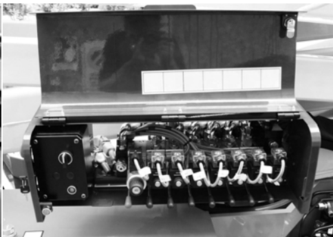
Fig. 64 Hydrauliske jordbetjeninger
