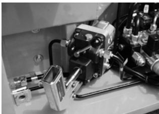
Fig. 70 Manual deviator til håndpumpe
